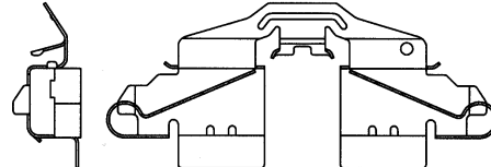
24309N and 24309Q – Pontiac, Toyota D1354, D1423 Quantity per wheel: 2
