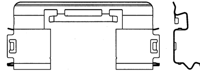
24357N and 24357Q – Cadillac D1422 Quantity per wheel 2
