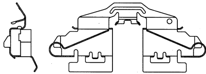
24308N and 24308Q – Pontiac, Toyota D1354, D1423 Quantity per wheel: 2
