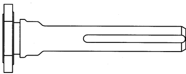
24285 – Dodge, D1399. Quantity per wheel: 2
