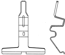
22671 – Mercedes Benz, D739, D779, D873, D876. Quantity per RH wheel: 1
