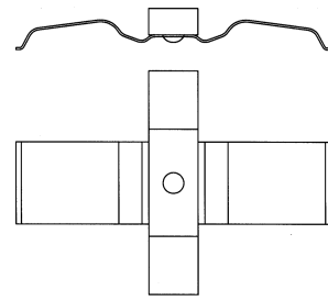
24283 – Infiniti, Nissan, D960. Quantity per wheel: 1
