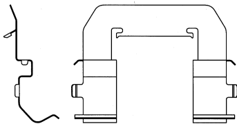
24320, 24320N & 24320Q – Chevrolet, D1404. Quantity per wheel: 2
