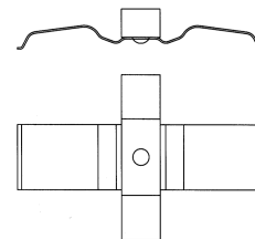
24276 – Mercedes Benz, D984. Quantity per wheel: 1
